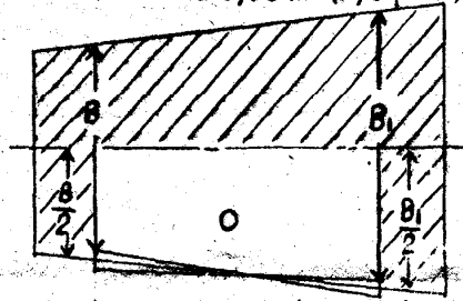
abertura en un solo costado
